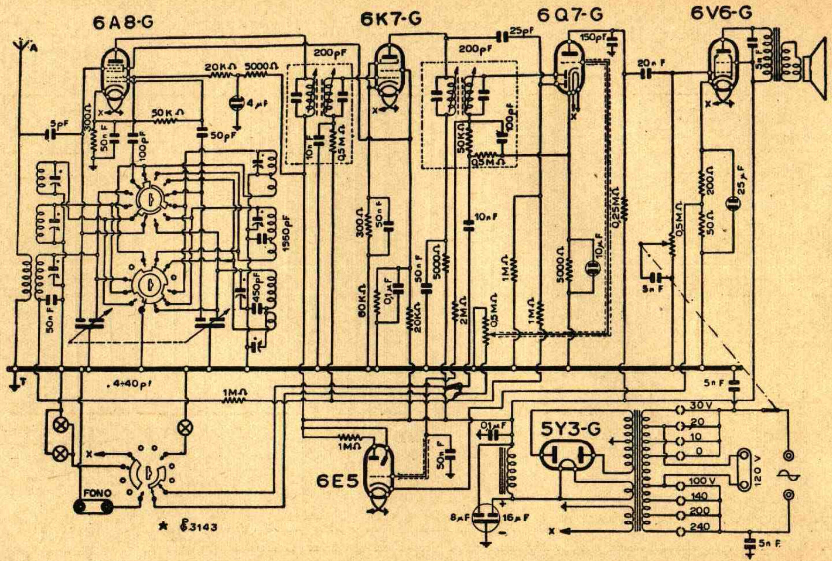
Lo schema elettrico dei modd. "528,, e "590,, Siare (telajo 2631).
